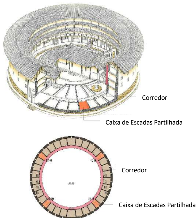
Figura 27 - Axonometria e planta esquemática de um tulou, adaptadas de Senses Atlas.
