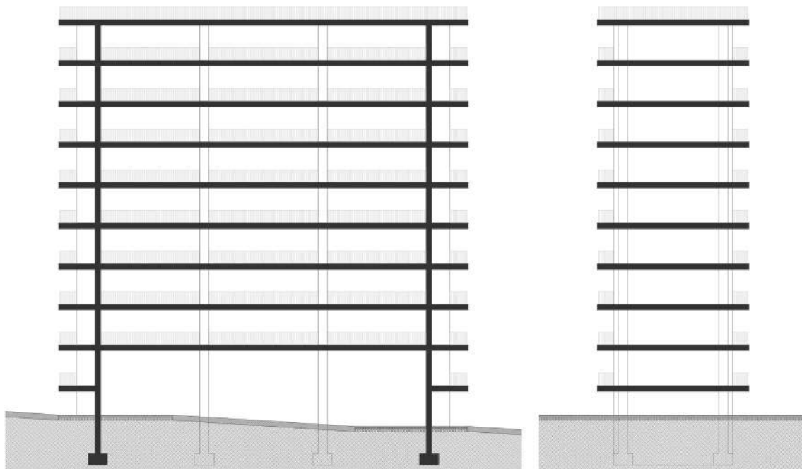
Figura 34 - Corte longitudinal e transversal.
