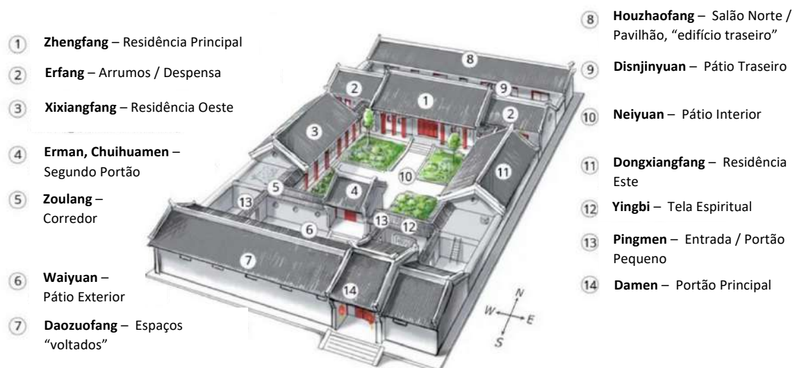
Fig. 24 - Axonometria esquemática de uma siheyuan , adaptada de China Highlights.
