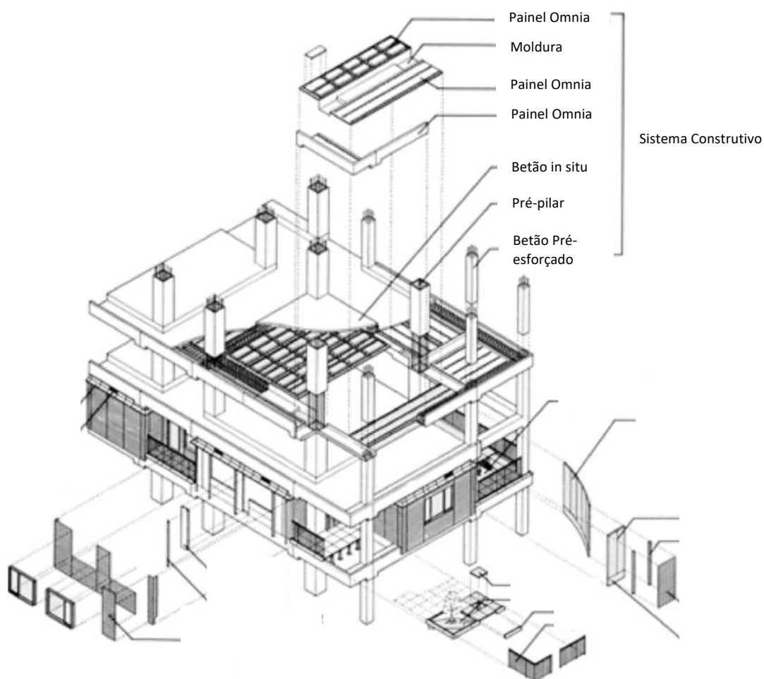
Figura 14 - Esquema do Sistema Construtivo do Edifício Next21, adaptado de The Council on Open Building ( https://councilonopenbuilding.org ).
