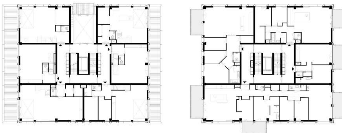
Figura 18 - Plantas de primeiro e segundo piso (respetivamente) de um edificio Sketchblock de Open Building.
