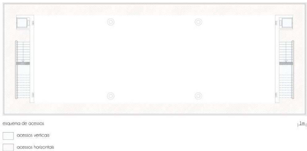
Figura 35 - Planta esquemática dos acessos verticais e horizontais dos pisos habitacionais.
