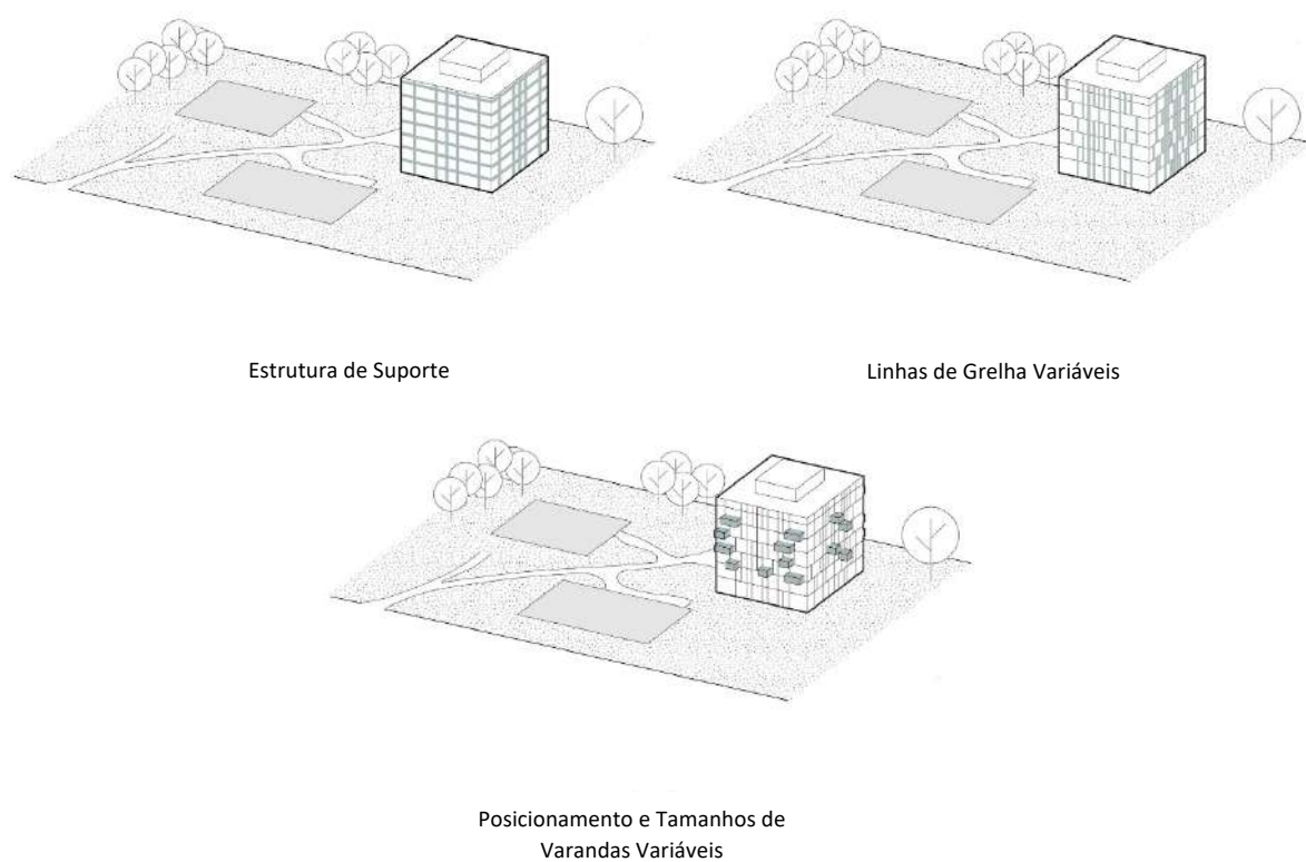
Figura 20 - Esquemas da flexibilidade das fachadas dos edifícios Sketchblock, adaptado de Open Building.
