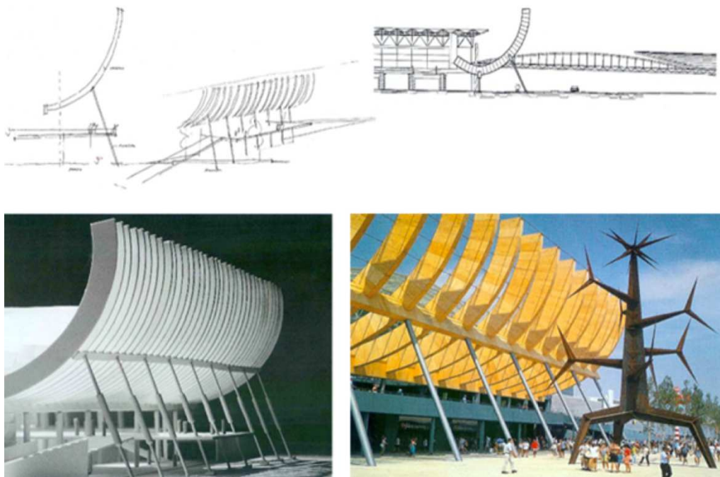
Figura 12 - Porta do Sol de Daciano da Costa
