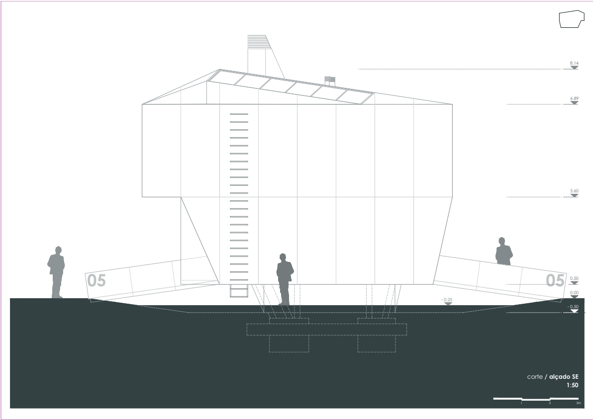
Sines 2015-2016. Casa e trabalho - Alçados. Paulo Peixoto (aluno)
