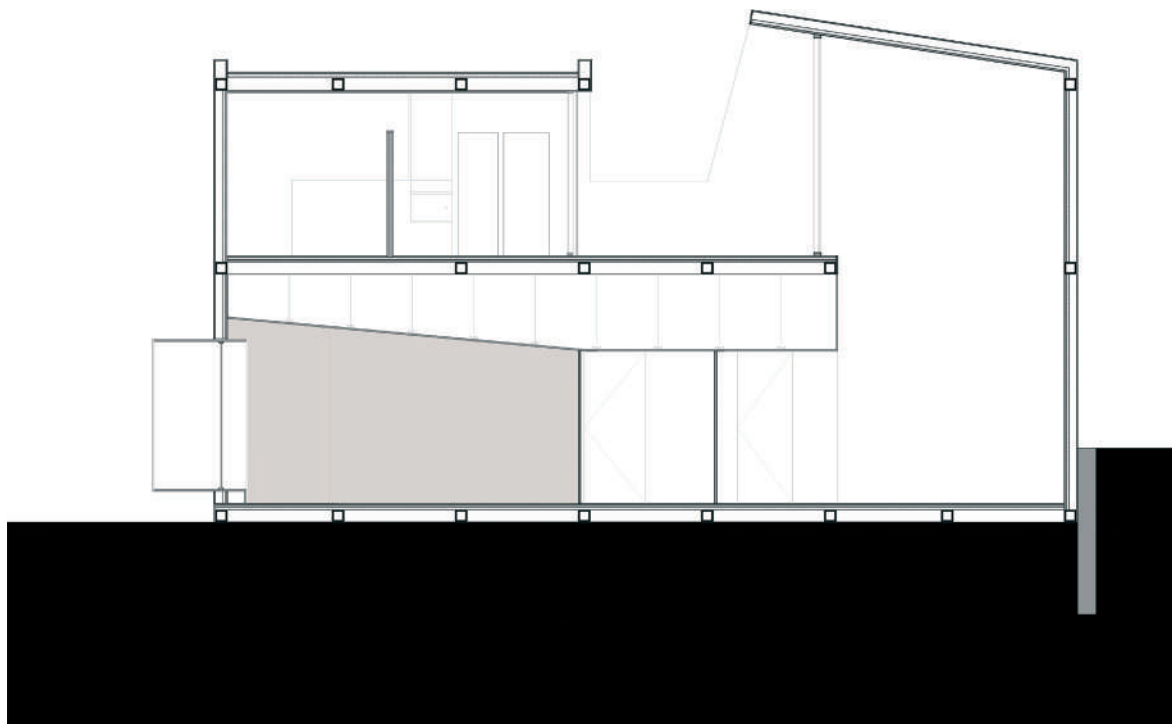
Campolide 2015-2016. Casa e trabalho - Tipologia com anexos 2. a versão - Planta e corte. Gonalo Vilhena (aluno)
