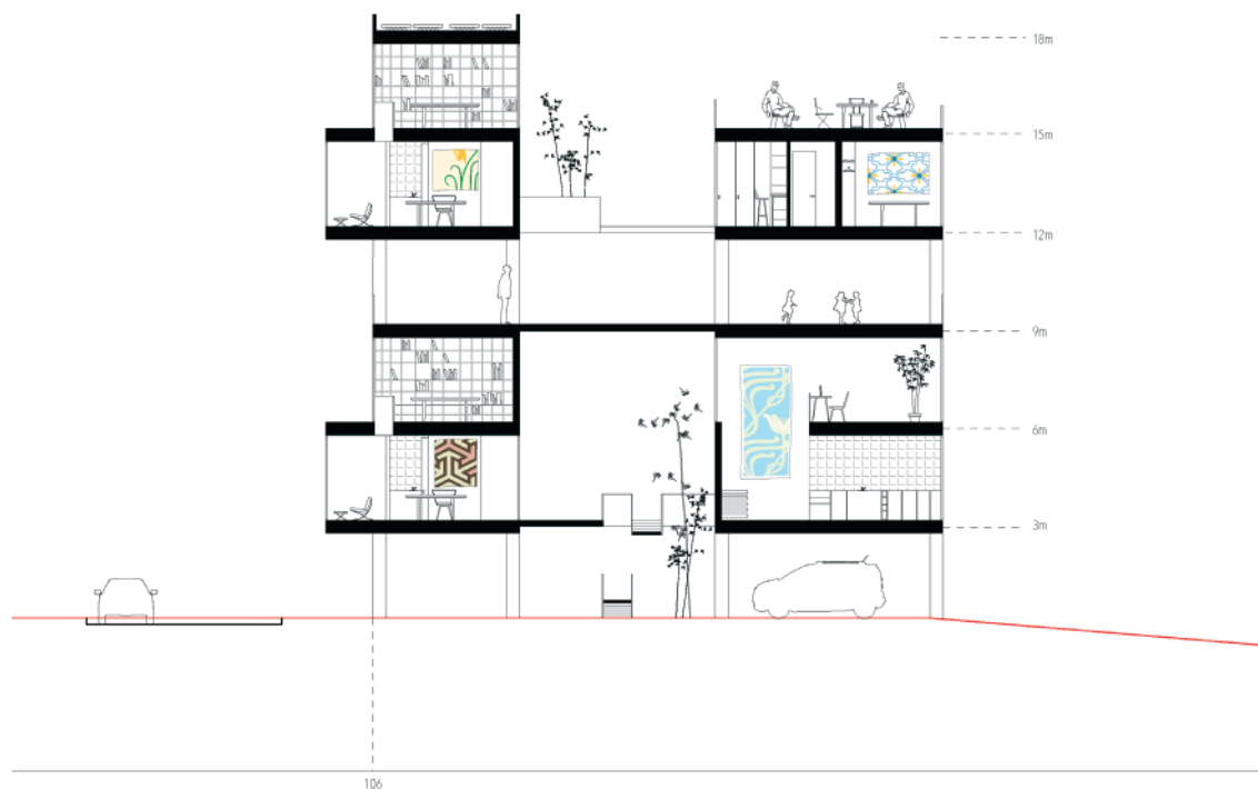
Alto dos Moinhos 2016-2017. Casa e trabalho - corte e volumetrias. Elvire Varine (aluna)
