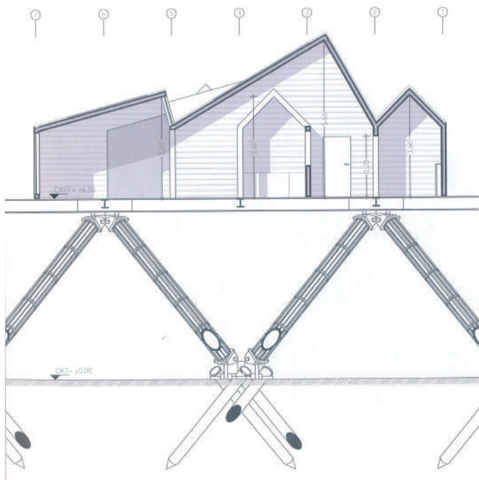
Sines 2015-2016. Casa e trabalho - estrutura e volumetrias. Andrea Fortunati e Aaron Leonard (alunos)
