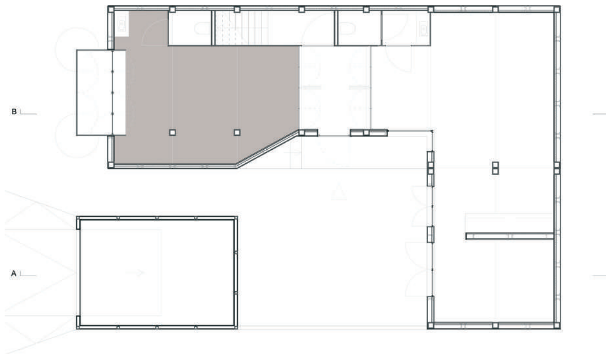
Campolide 2015-2016. Casa e trabalho - Tipologia com anexos 2. a versão - Planta e corte. Gonalo Vilhena (aluno)
