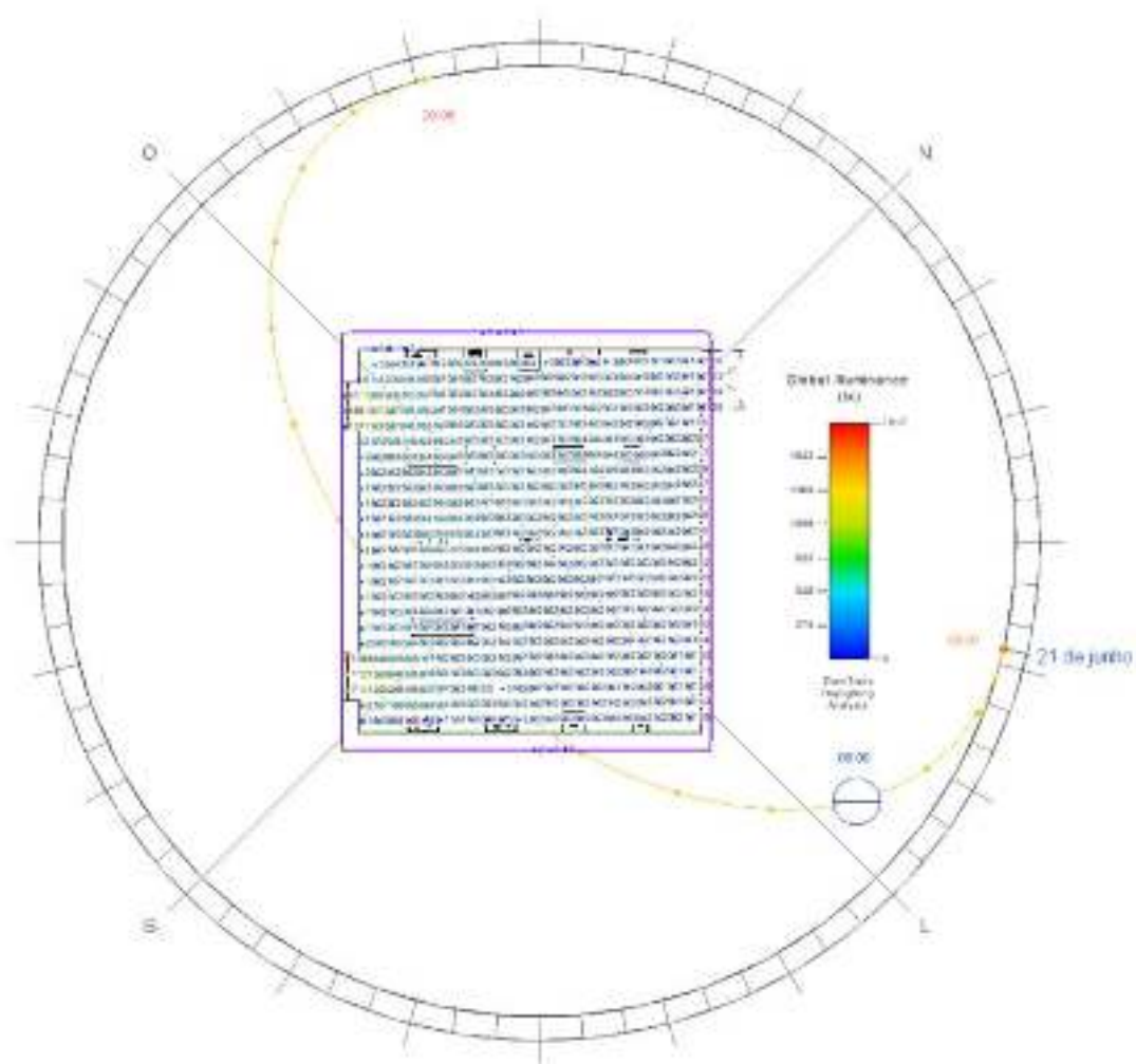
Fig. 110A - Iluminância nos pontos da grelha para o Cenário AN2 no solstício de verão às 08h00.
