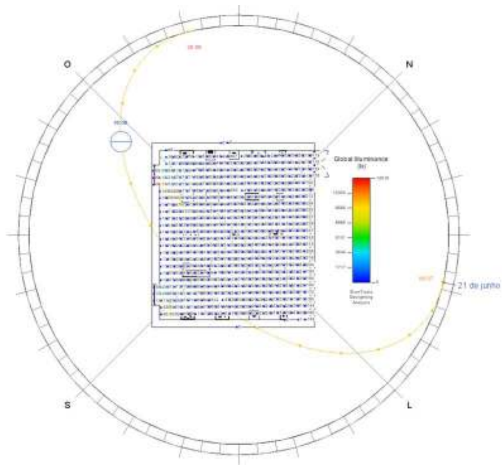
Fig. 102A - Iluminância nos pontos da grelha para o Cenário AN1 no solstício de verão às 16h00.
