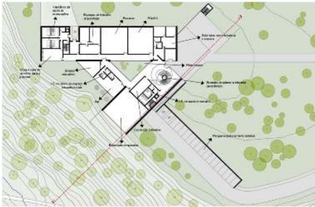
Fig. 45 – Planta piso 1.
