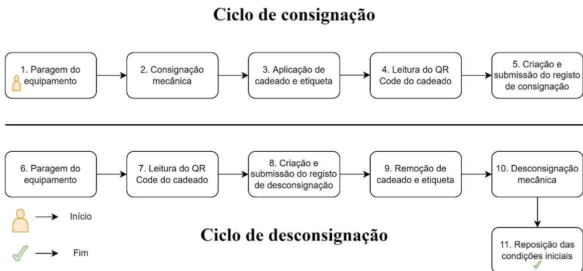
Figura 27 - Diagrama de processos para o procedimento LOTO de processo de consignação e desconsignação mecânico (processo especial).
