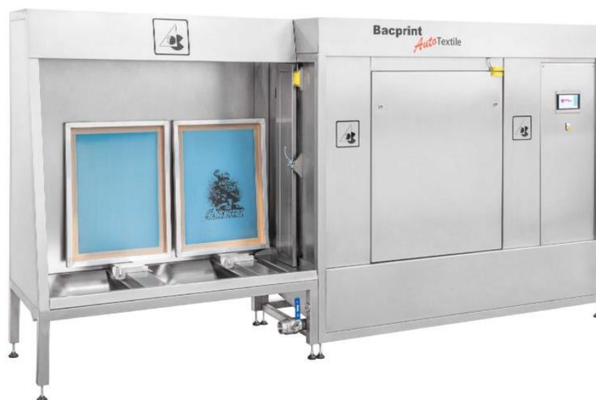
Figura 41. Equipamento proposto para limpeza, Bacprint auto textile (Acosgraf, 2019).
