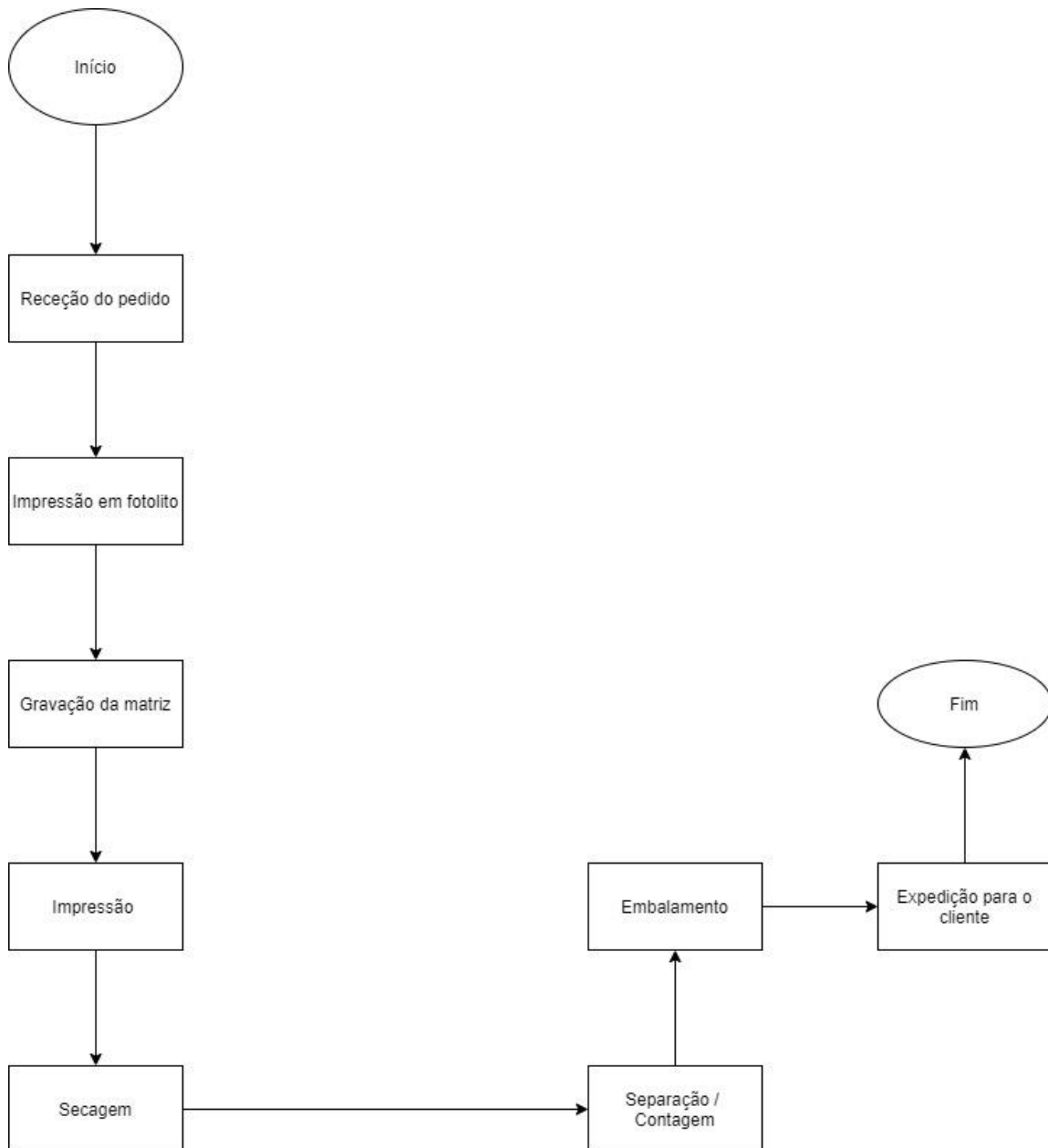
Figura 18. Fluxograma do processo produtivo de autocolantes.
