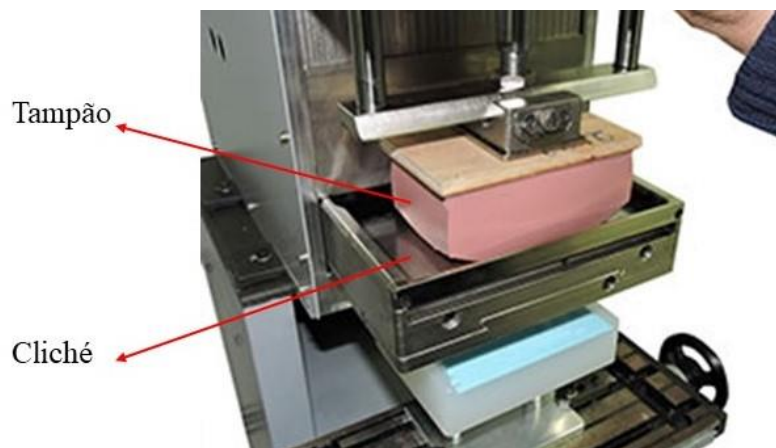
Figura 22. Cliché e tampão colocados na máquina de impressão (adaptado de Flues, 2015).
