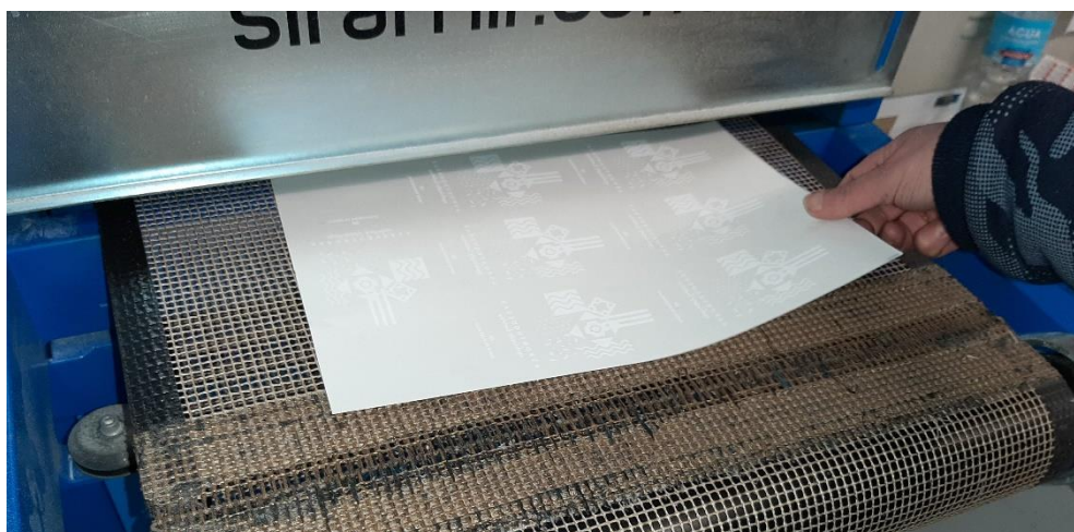
Figura 29. Entrada do plano com transfers no túnel de secagem.
