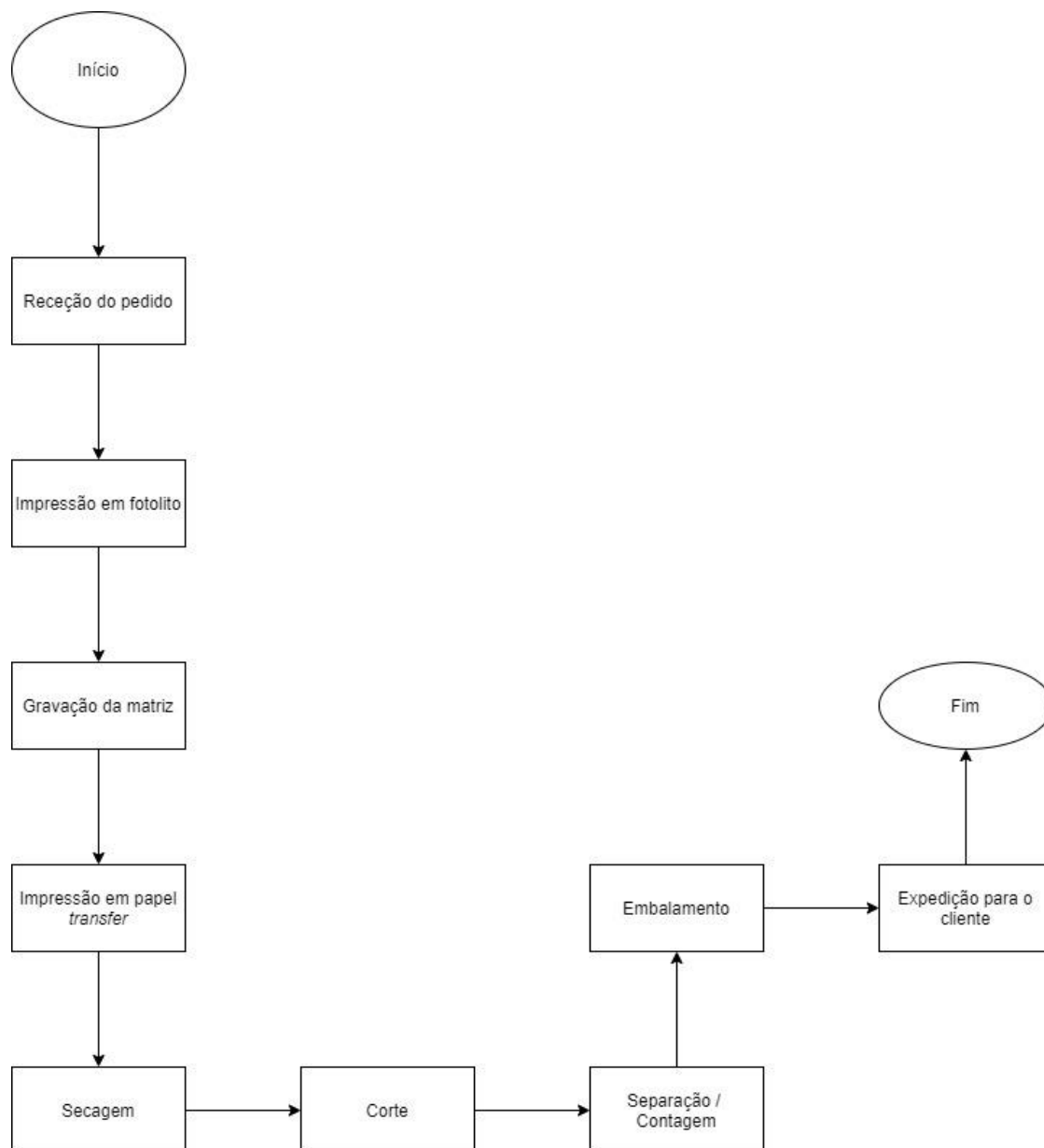
Figura 14. Fluxograma do processo produtivo de transfers .
