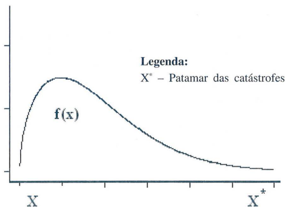
Figura 1 – Função de densidade
