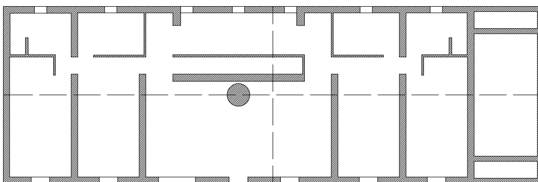
Ilustração 57 - Diagrama de eixos, piso térreo casa de Blas (Ilustração nossa, 2018).
