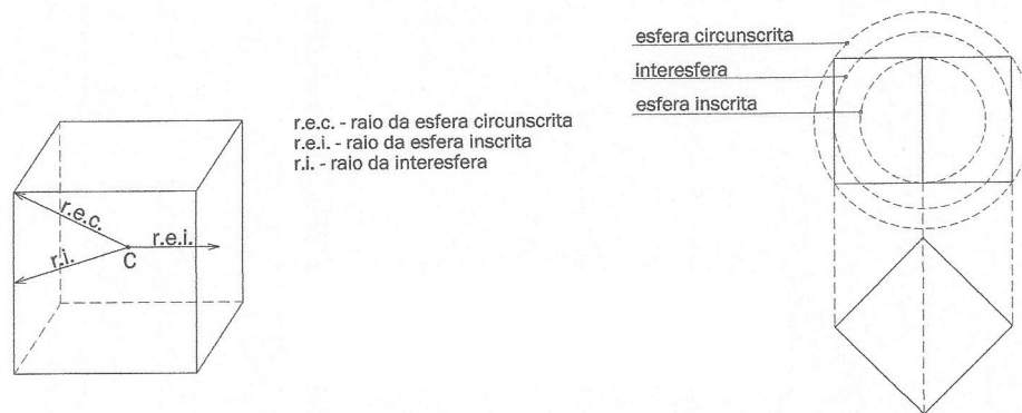
Fig. 6 - As distâncias do centro do sólido às faces e aos vértices correspondem aos raios das esferas inscrita e circunscrita.
