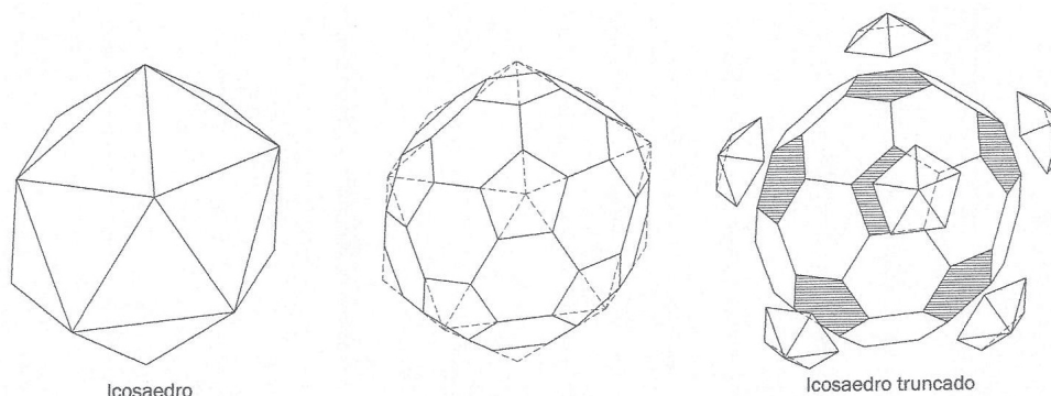
Fig. 14 - Obtenção do icosaedro truncado a partir do icosaedro.
