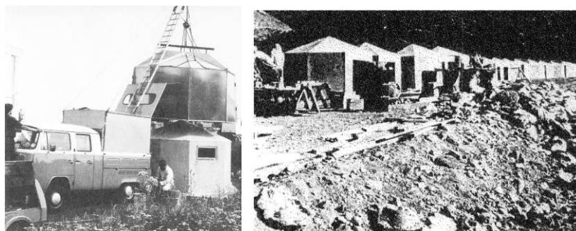
Figura 23- Iglôs hexagonais utilizados pela UNDRO no decorrer no terramoto em Lice, Turquia, em 1975
